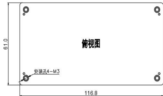
标准型 116.8*61*12.7mm
