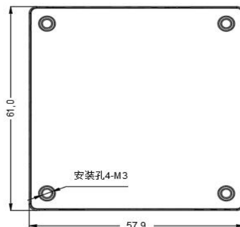
标准型 61.0*57.9*12.7mm
