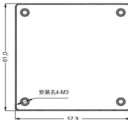
标准型 61.0*57.9*12.7mm
