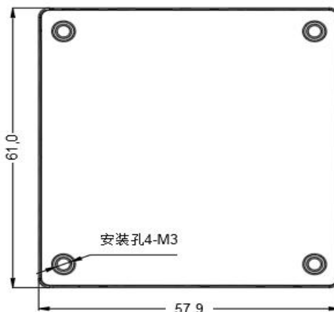
标准型 61.0*57.9*12.7mm
